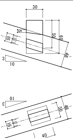
側面図による A,B,C 貫詳細図
