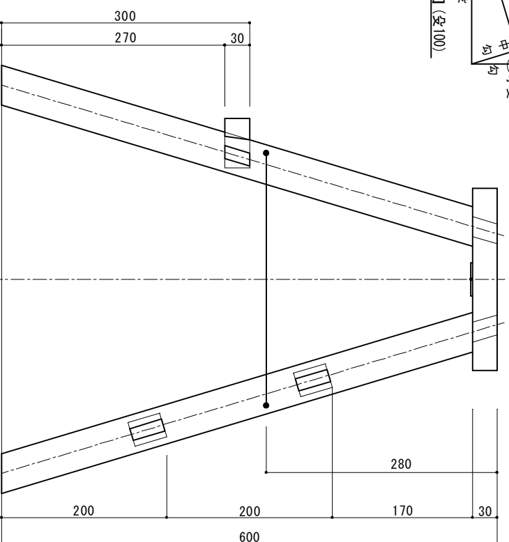
側面図
