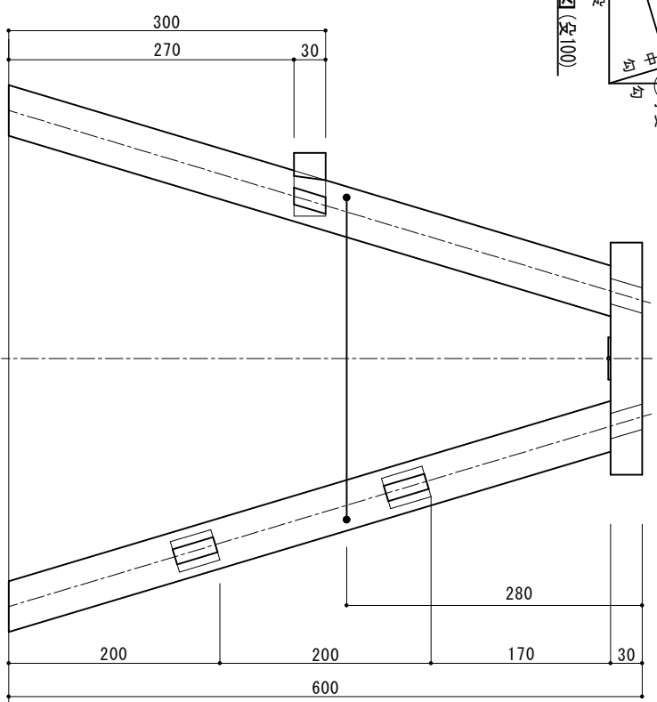
側面図
