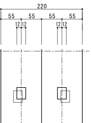
天板平面图
