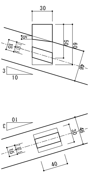
側面図による A, B, C 貫詳細図
